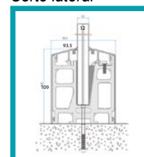
Corte lateral
