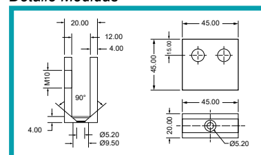
Detalle Medidas
